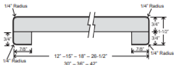
BAR TOP CNB 12 CNB 15 CNB 18 CNB 26-1/2 CNB 30 CNB 36 CNB 42
