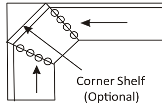
22 1/2" Mitres: (Provide template)
