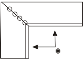
Reverse Mitres: * (Provide wall Dim.)
